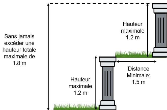
Figure 6 – Mur de soutènement
